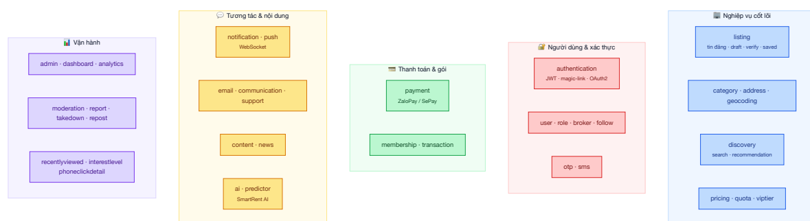
Hình 3.5: Các module nghiệp vụ của Backend gom theo cụm chức năng
