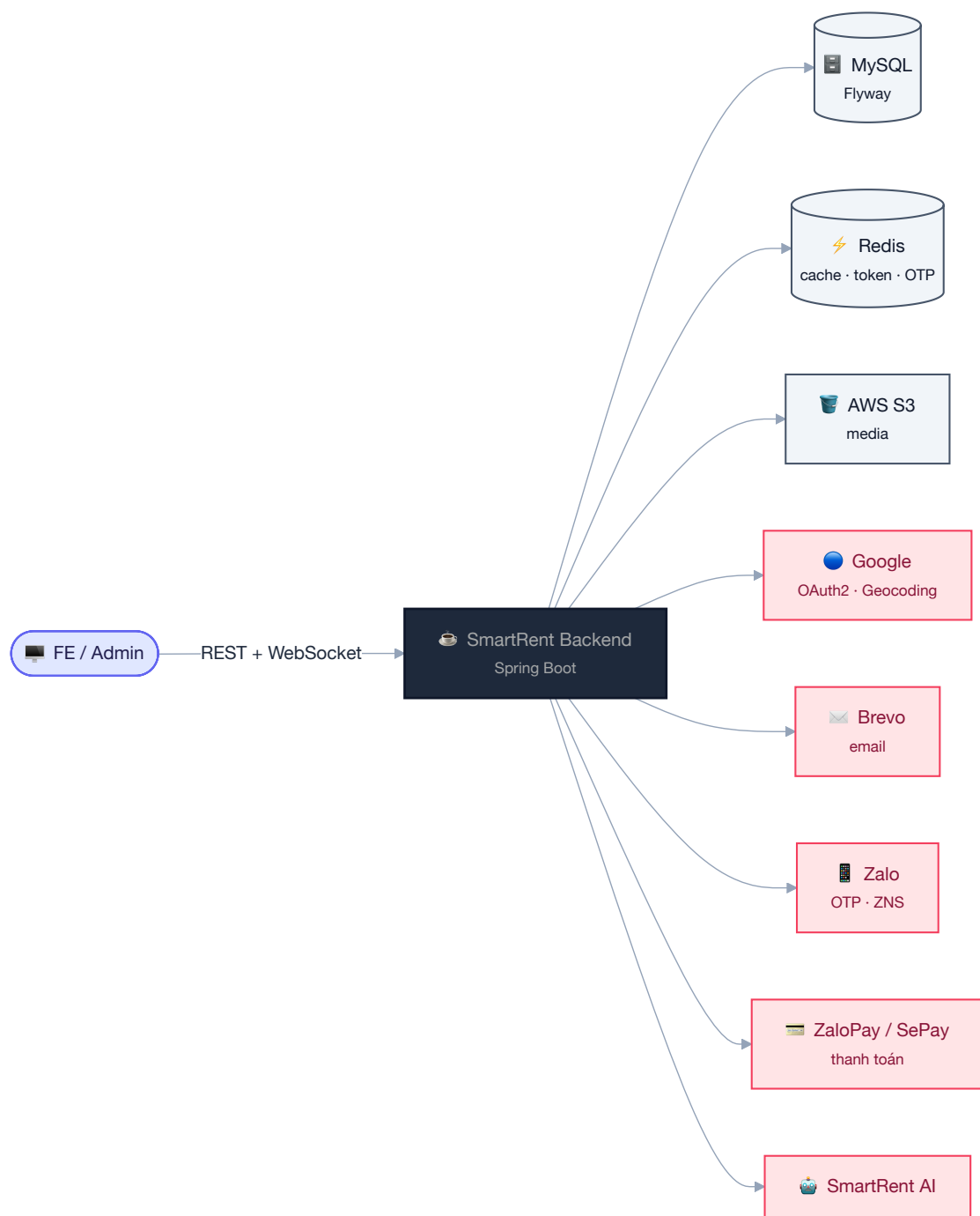
Hình 3.4: Các dịch vụ bên ngoài mà Backend tích hợp
