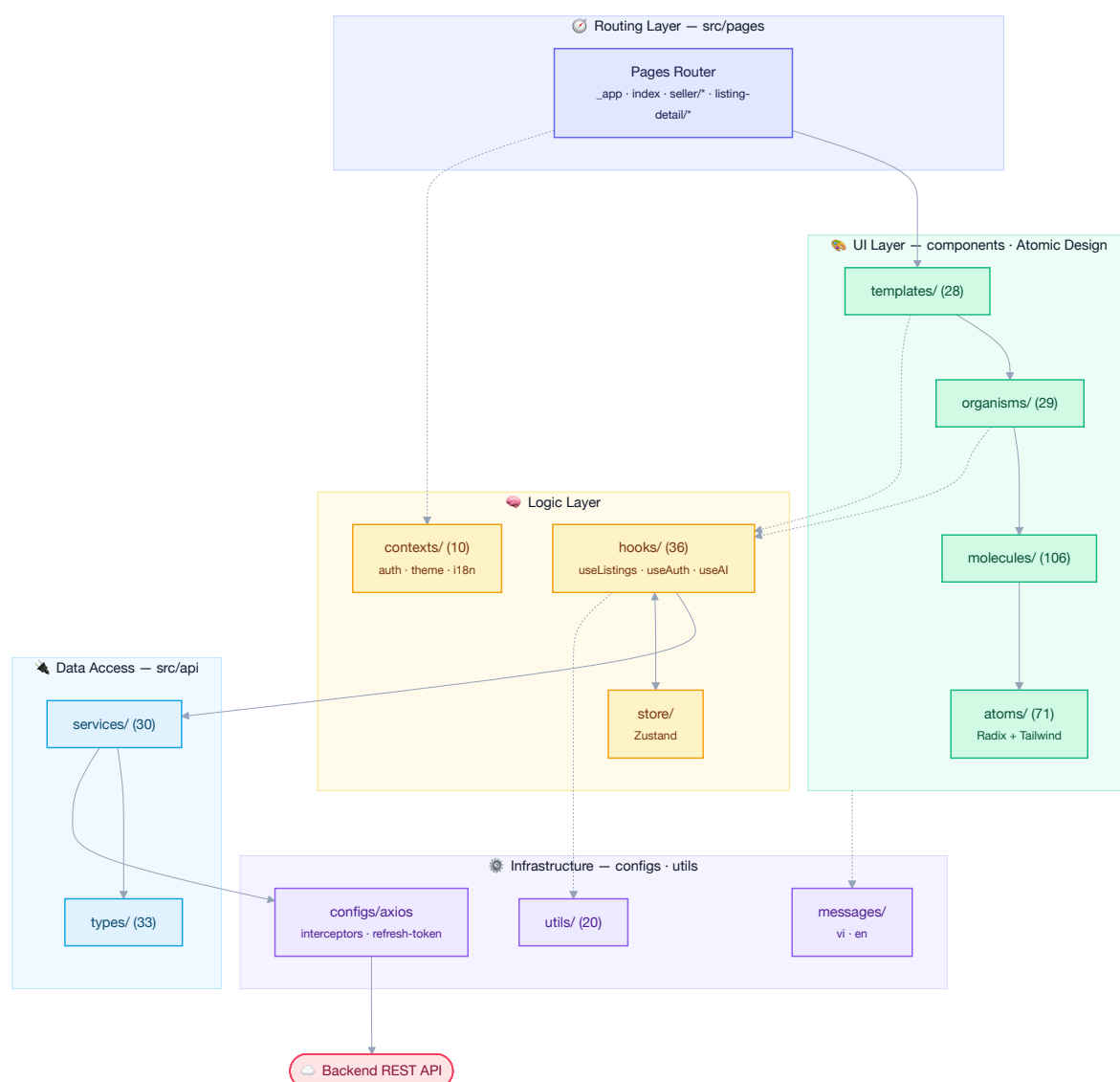
Hình 3.1: Sơ đồ tổ chức mã nguồn ứng dụng web (webapp)
