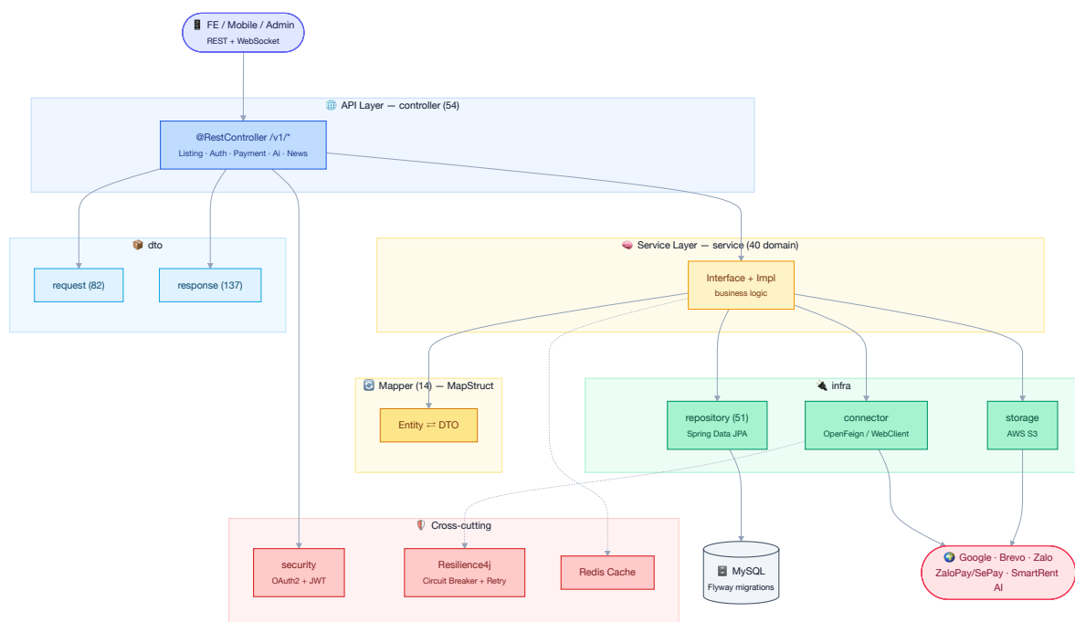
Hình 3.3: Kiến trúc phân lớp của hệ thống Backend (Modular Monolith)
