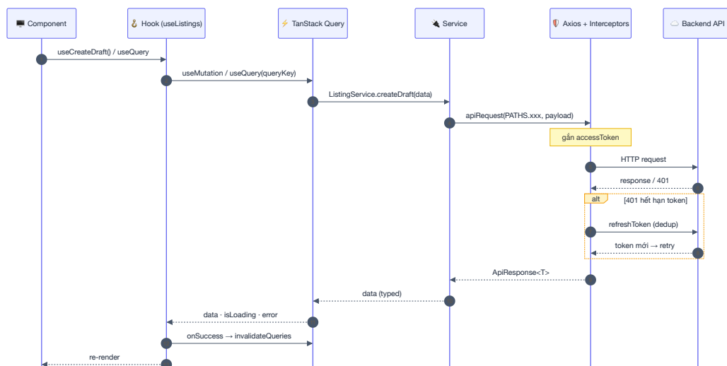
Hình 3.2: Luồng dữ liệu giữa giao diện, hook, tầng dịch vụ và Backend
