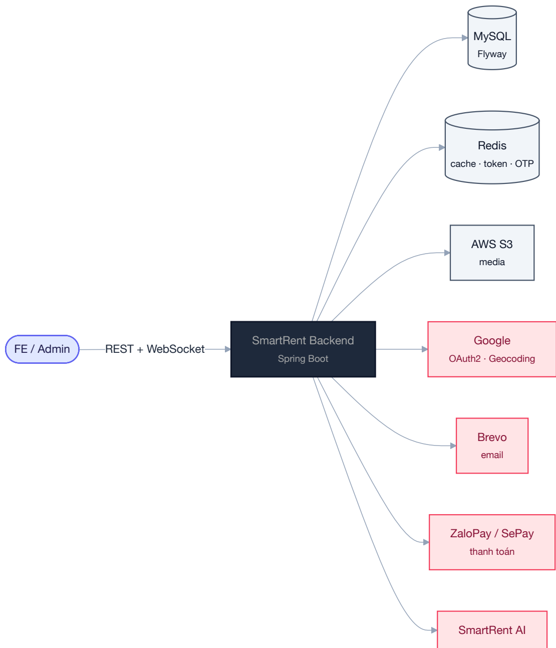
Hình 4.4: Các dịch vụ bên ngoài mà Backend tích hợp
