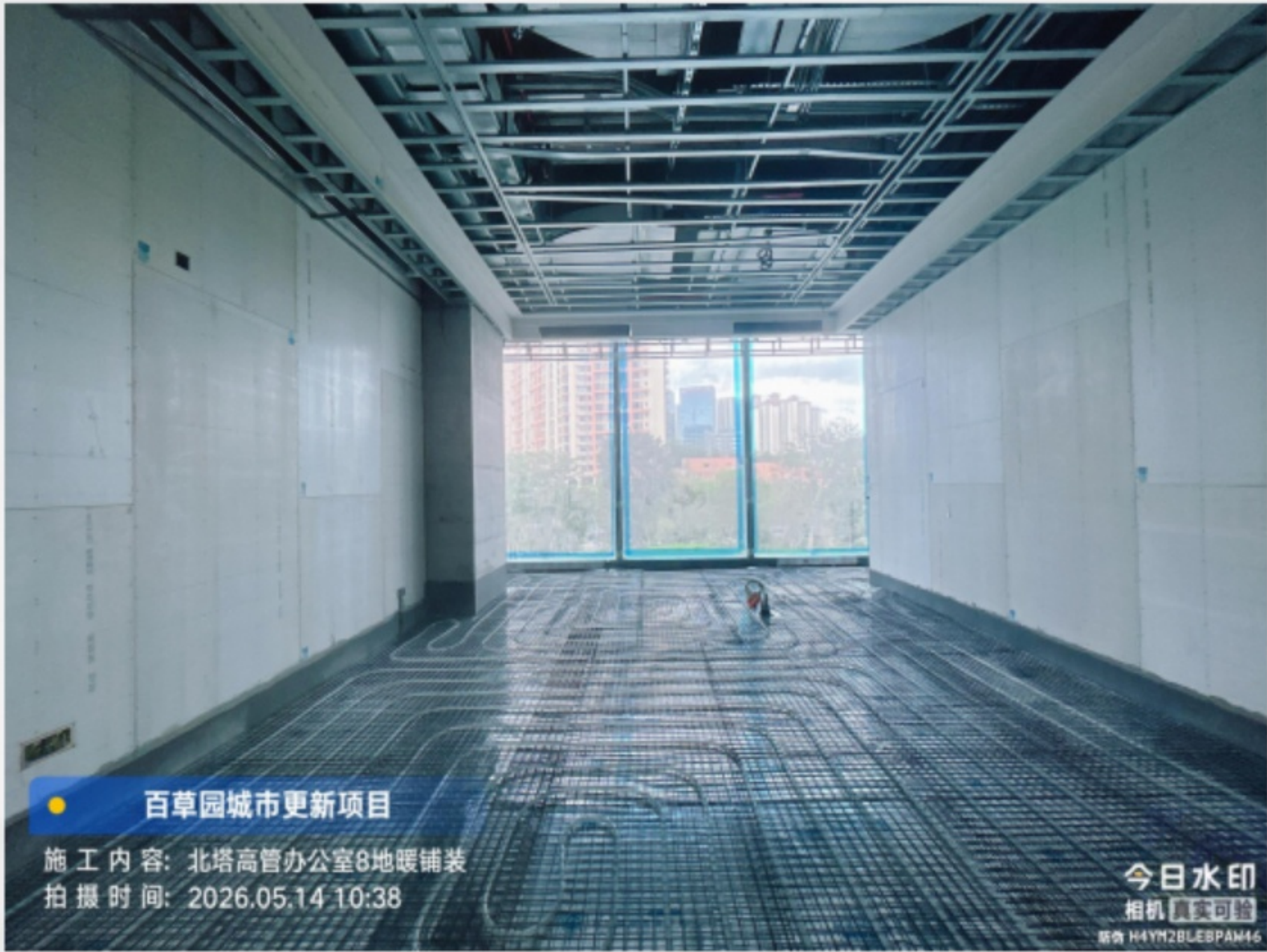
高管办公区8层地暖铺装施工，地面钢筋网片已铺设完成
