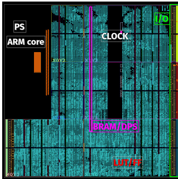
Zynq-7000 SoC
