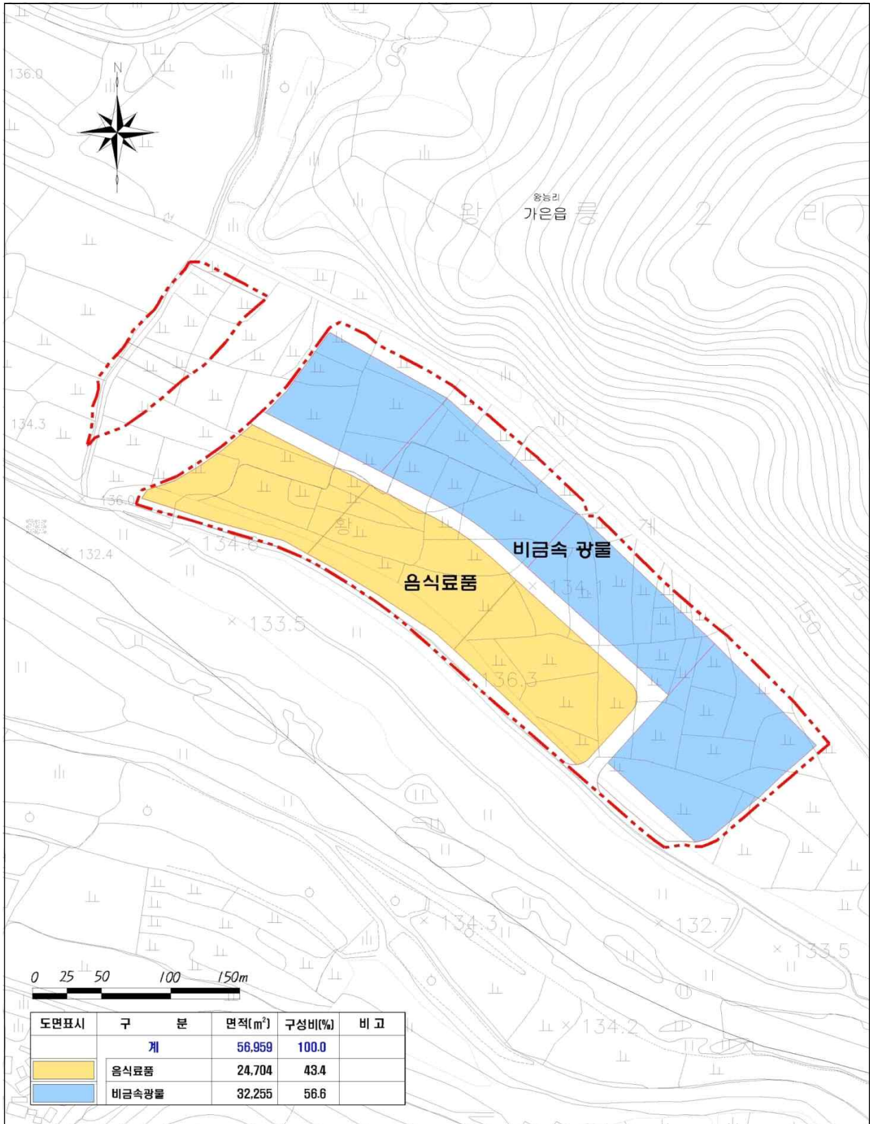
【별표3】 업종별 배치계획도
