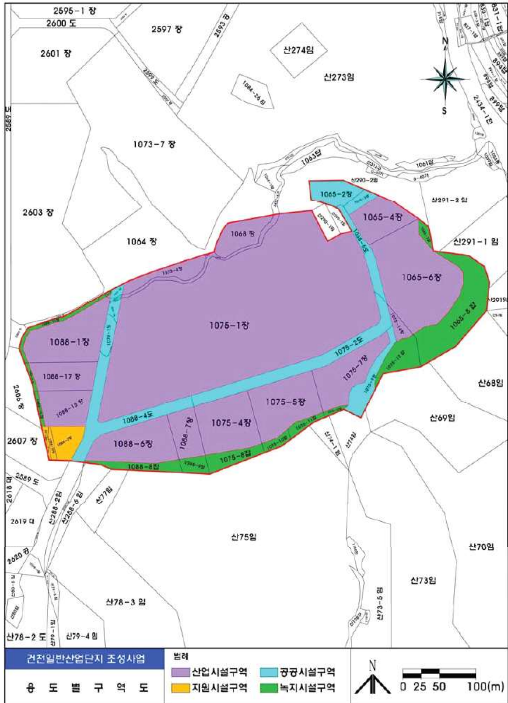
별표 1 : 용도별 구역도
