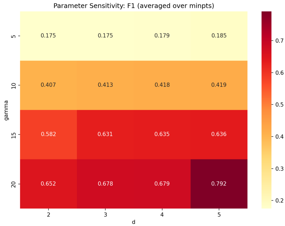
Figure 5: 파라미터 민감도 — \gamma \times d 파라미터 조합별 F1. 171 가지 가중치 조합 중 71.9% 에서 MutClust-Hybrid 1 위 유지.
