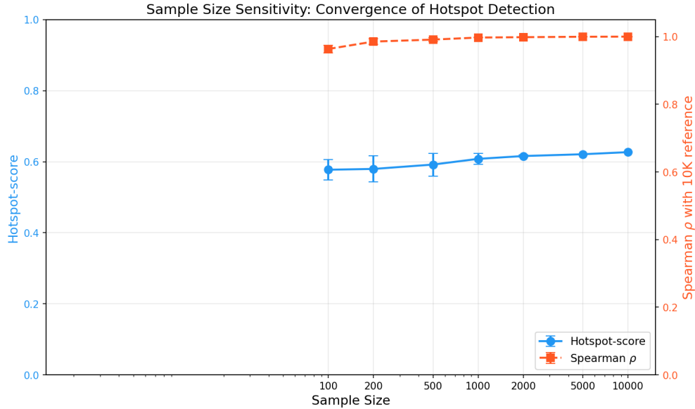
Figure 4: 표본 크기 수렴 — 약 1,000 개 서열부터 hotspot-score 약 0.62 로 안정화. 본 벤치마크 서열 수 (662~5,325) 는 수렴점 이상.
