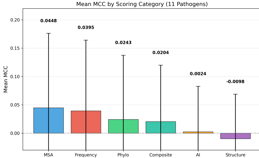
Figure 7: Scoring 카테고리별 평균 MCC (11 병원체). 빈도 기반과 MSA 파생이 평균적으로 높으나 오차 막대가 크므로 카테고리 수준 일반화는 불충분.
