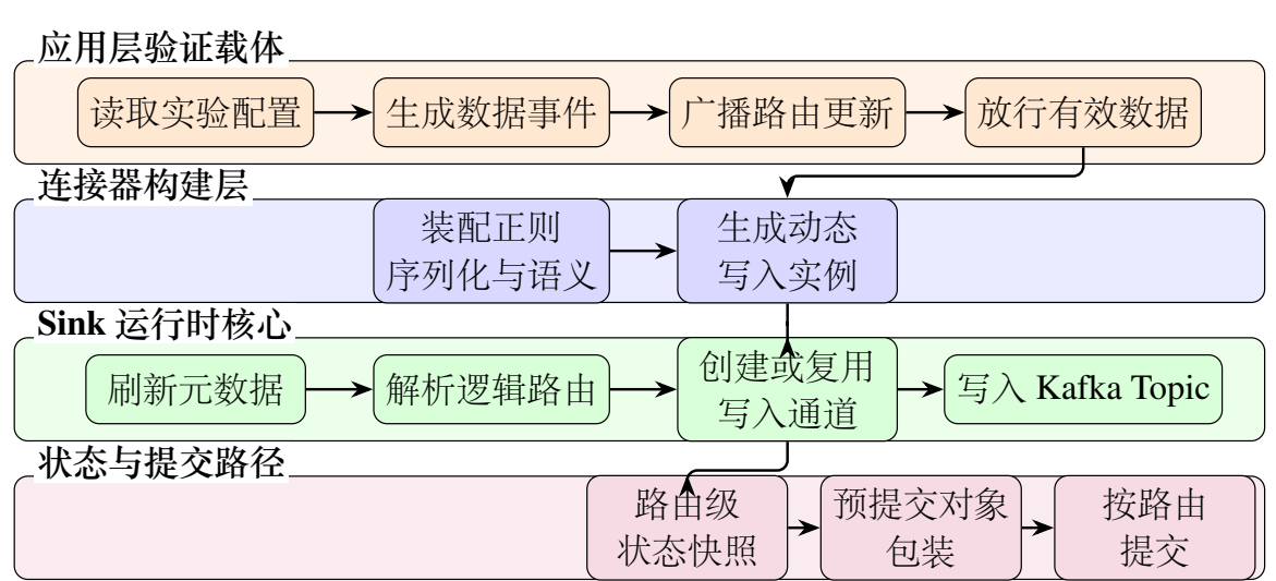
图 4-2 动态 Sink 分层调用关系与状态提交路径
