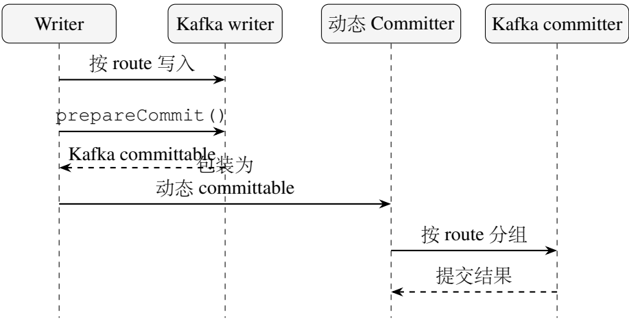
图 4-4 Exactly-once route 级提交流程序列图
