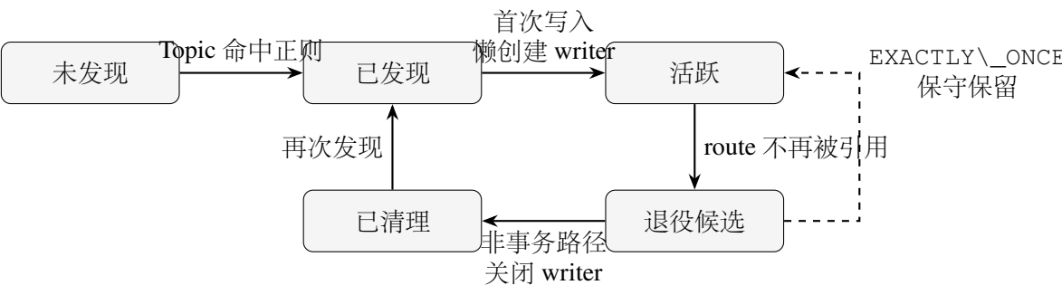
图 4-3 route 生命周期状态转移图
