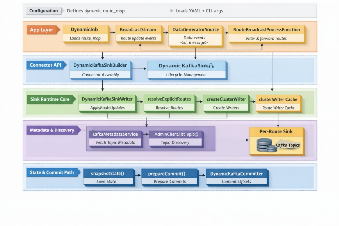
图 4-2 动态 Sink 分层调用关系与状态提交路径
