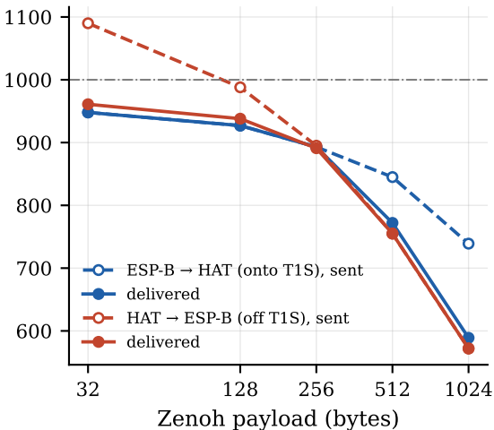
(b) message rate (dash-dot: 1000/s)
