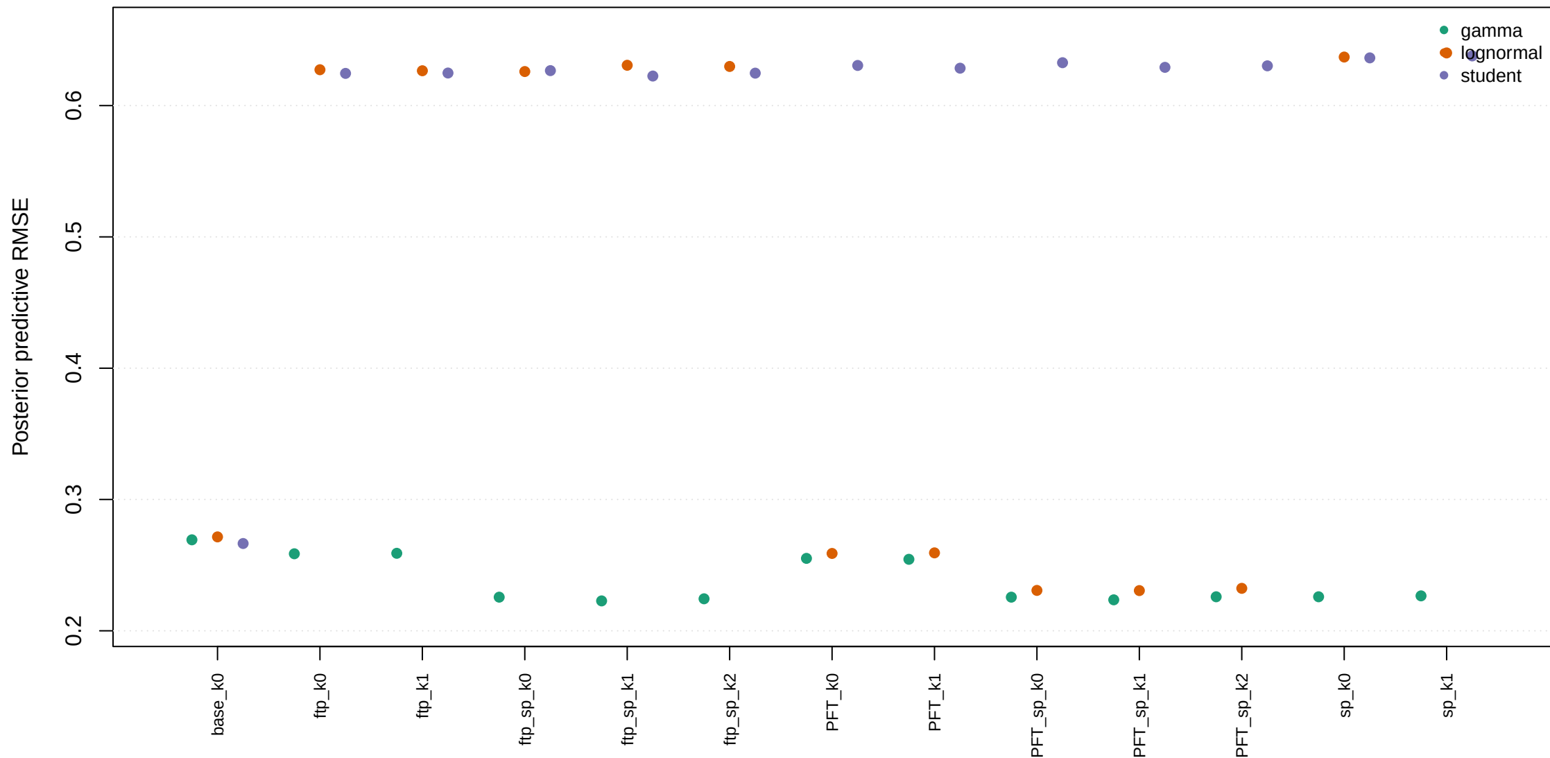
Posterior predictive RMSE: befr.st
