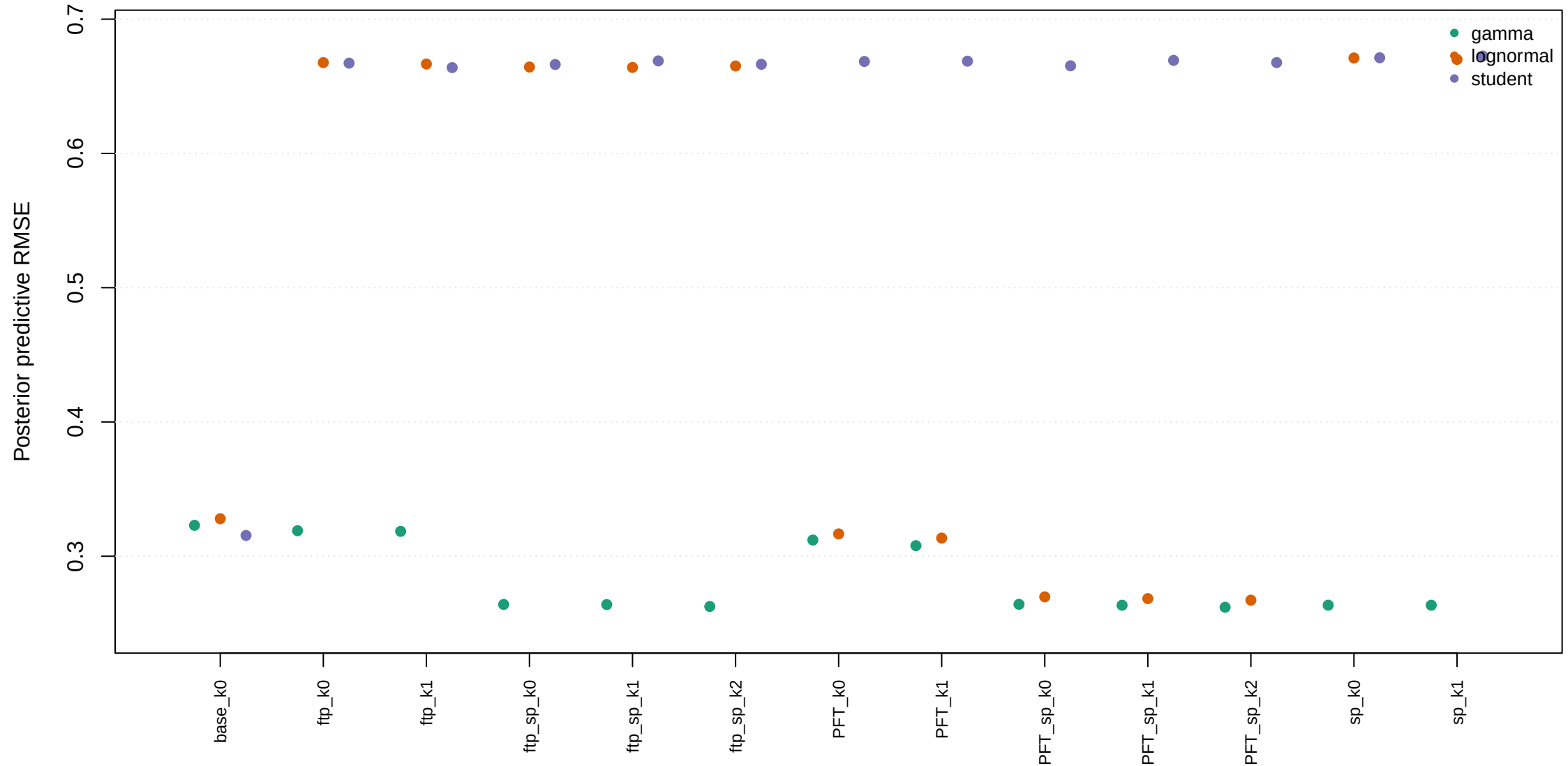
Posterior predictive RMSE: befa.st
