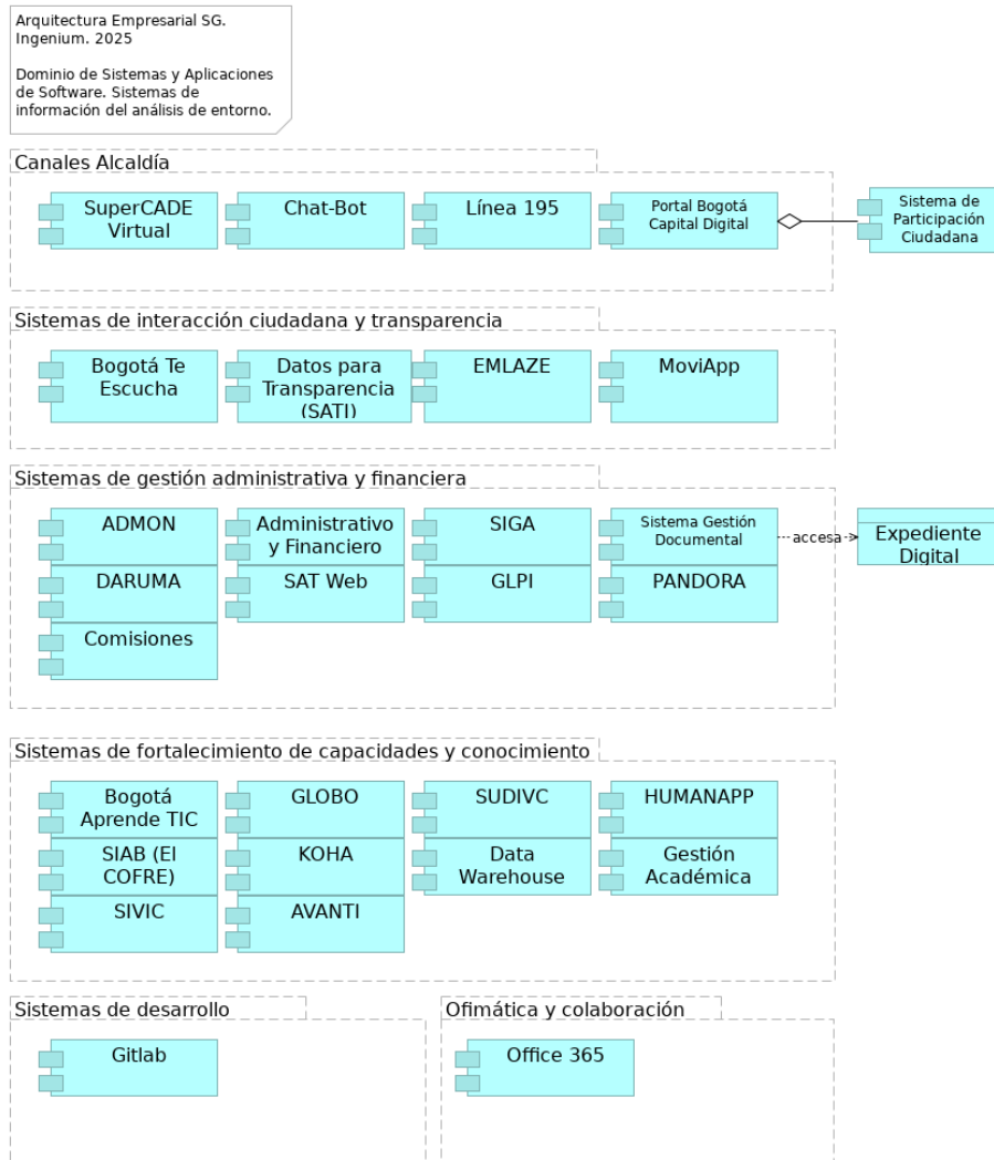
Figura 1: 06.2n2. SI del Analisis de Entorno. Fuente: Propuesta servicios de ingeniería y evaluación de arquitectura Arquitectura de Aplicaciones Secretaria de la Alcaldía de Bogotá (2025)
