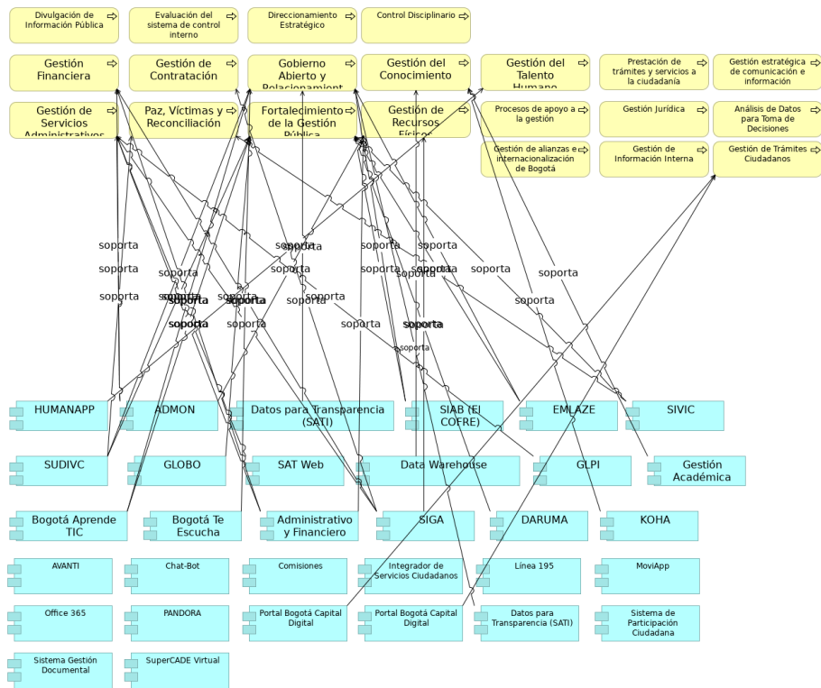
Figura 2: 06.2n3.a.Aplicaciones y Procesos. Fuente: Propuesta servicios de ingeniería y evaluación de arquitectura Arquitectura de Aplicaciones Secretaria de la Alcaldía de Bogotá (2025)
