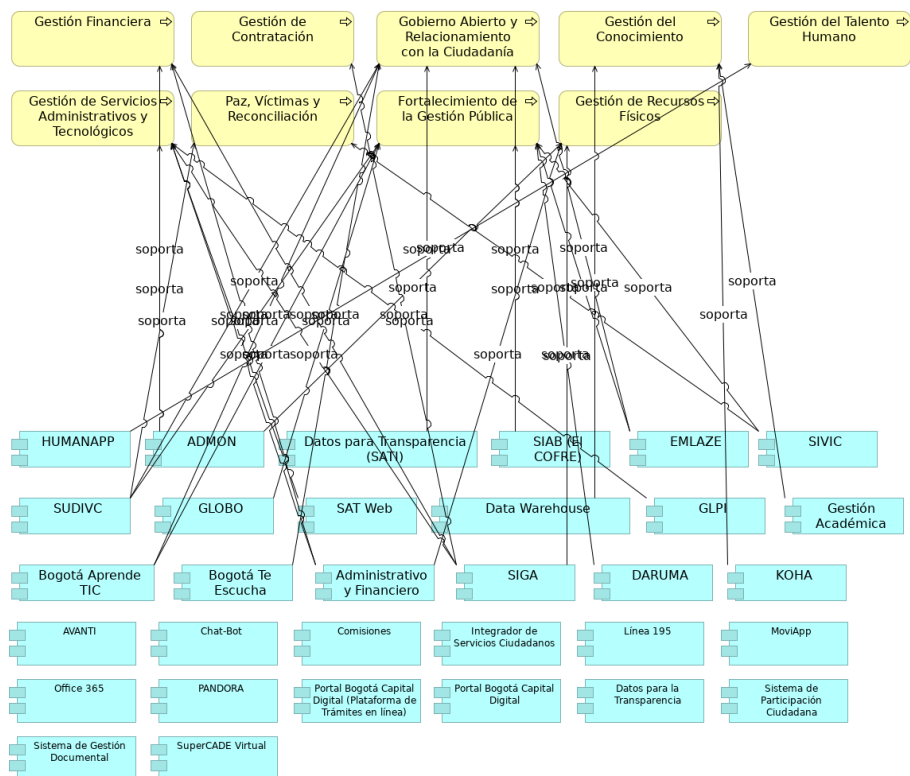
Figura 2: 06.2n3. Aplicación. Aplc y Procesos. Fuente: Propuesta servicios de ingeniería y evaluación de arquitectura Arquitectura de Aplicaciones Secretaria de la Alcaldía de Bogotá (2025)
