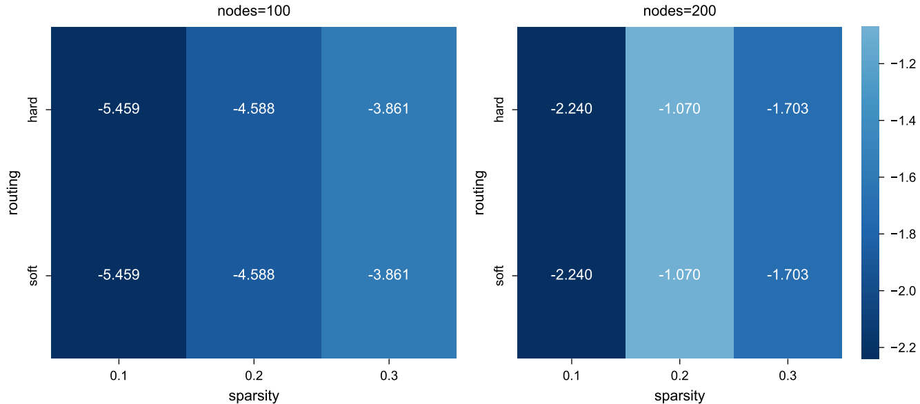
F4. Prior Effect Map (ETTh1 MSE, prior_true - prior_false)
