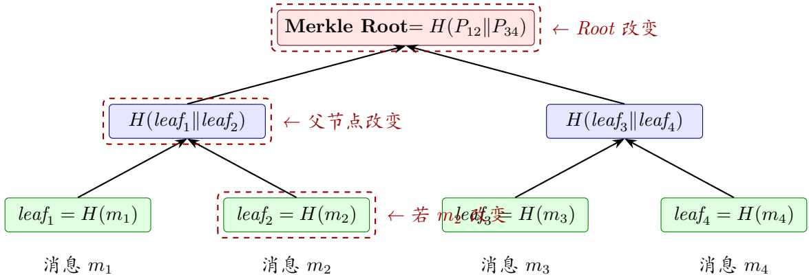
图 5: Merkle Tree 结构示意图（任意叶子变化均导致 Root 改变）
