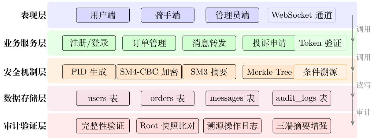
图 7: FoodShield 系统总体架构分层图
