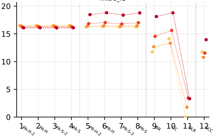
micro_f1
