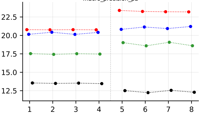
macro_precision_pa
