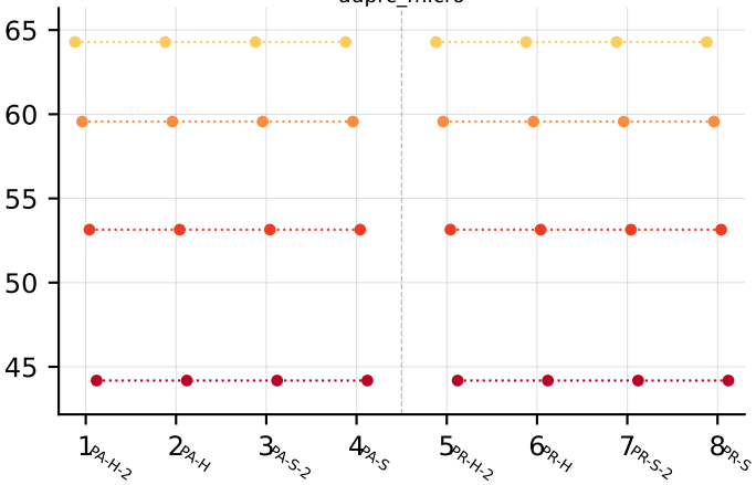
auprc_micro
