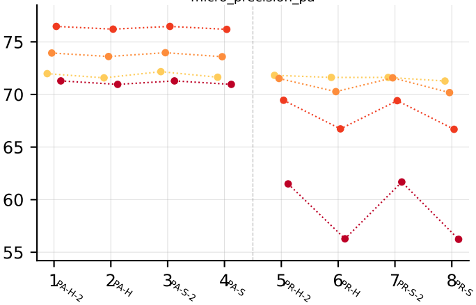
micro_precision_pa
