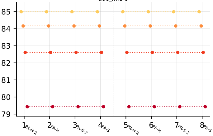
auc_micro
