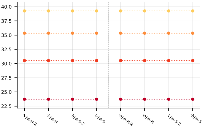
auprc_micro
