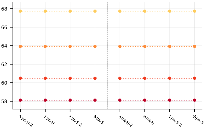
auc_macro
