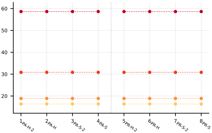
one_error
