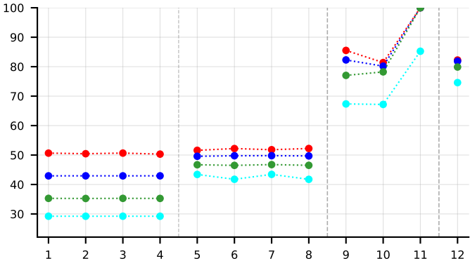
micro_precision
