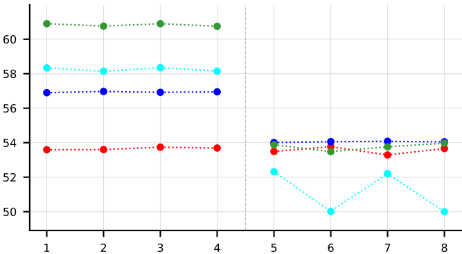
macro_f1_pa
