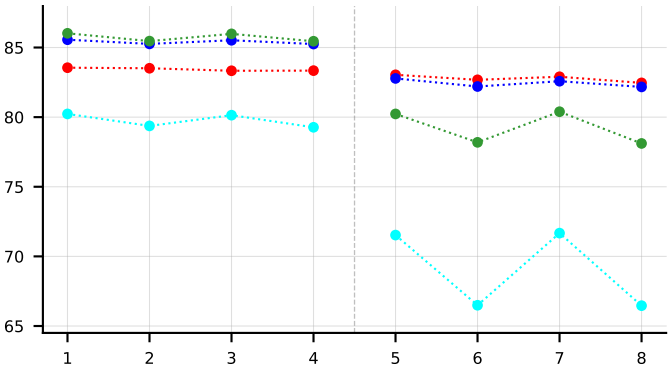
micro_f1_pa
