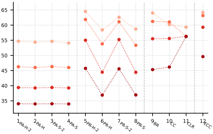
macro_precision
