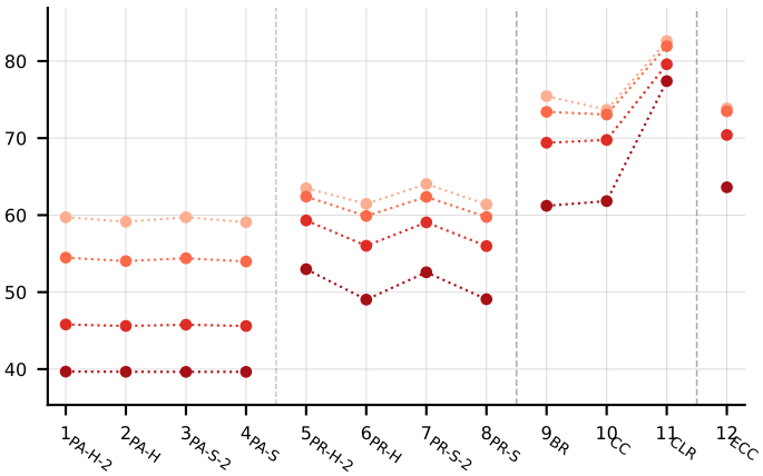
micro_precision
