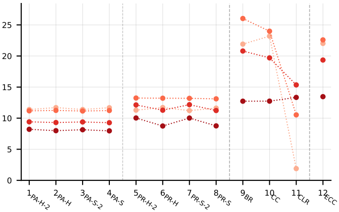
macro_f1
