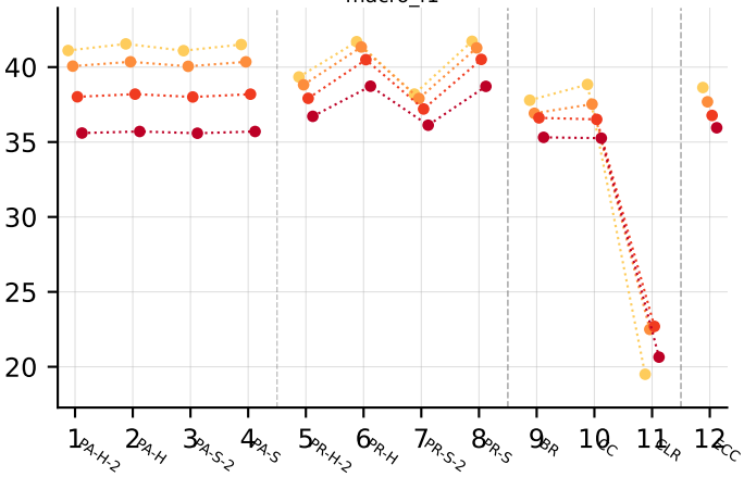
macro_f1
