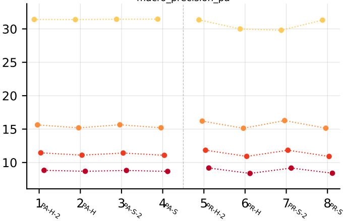
macro_precision_pa
