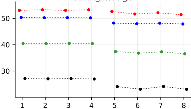
example_precision_pa
