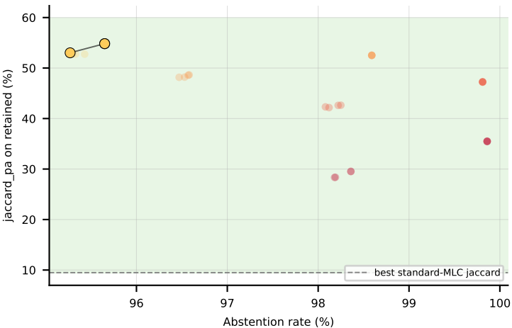
RF on HumanPseAAC (jaccard_pa) -- Pareto frontier + win-region
