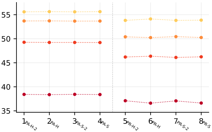
f1_pa
