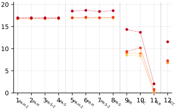
micro_f1
