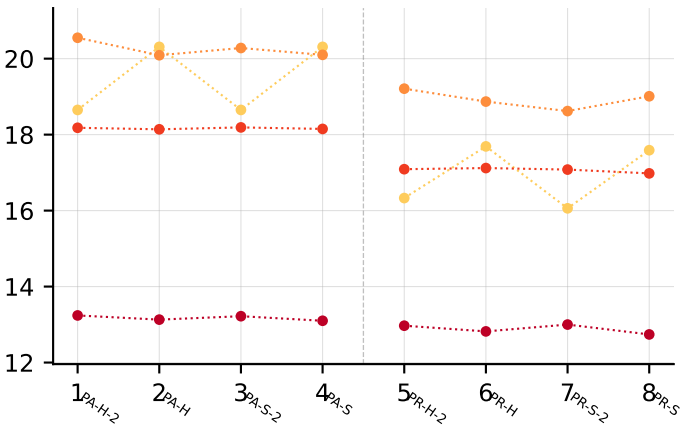
macro_precision_pa
