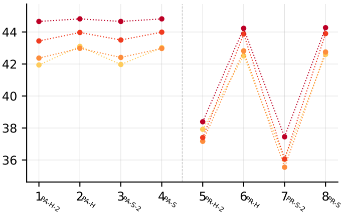
macro_f1_pa
