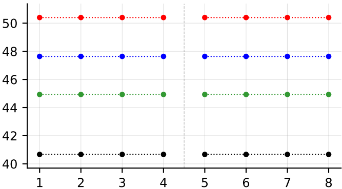
auprc_macro
