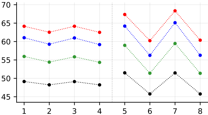
micro_precision_pa
