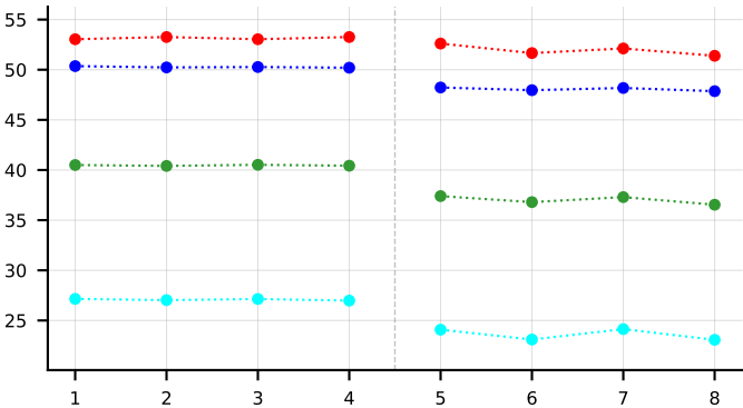
example_precision_pa
