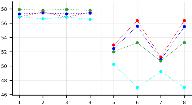
jaccard_pa
