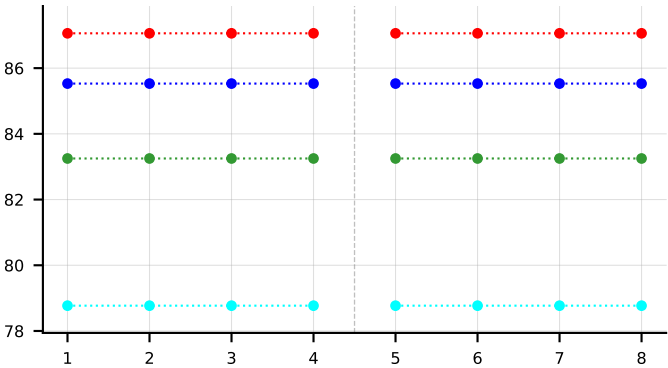
auc_micro
