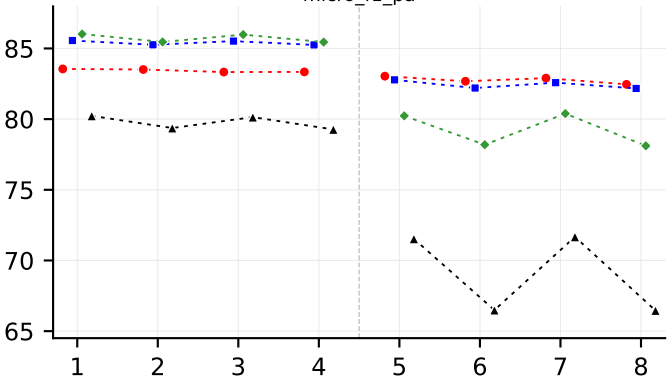
micro_f1_pa
