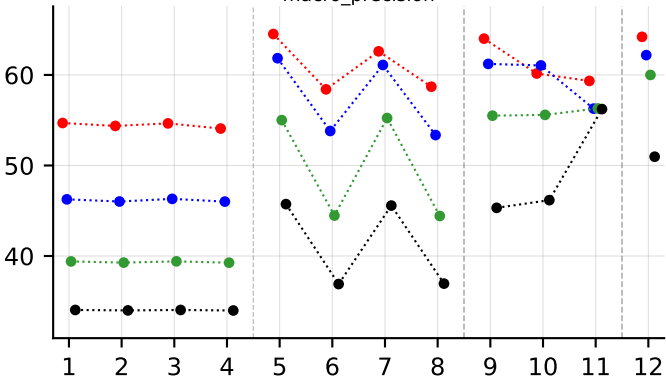
macro_precision
