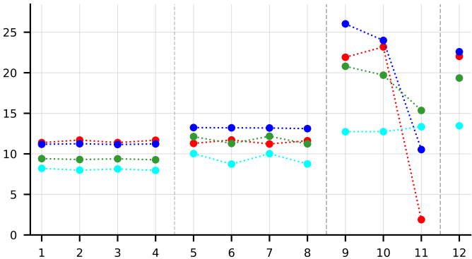
macro_f1
