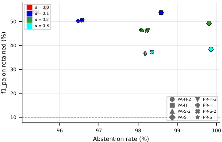
RF on HumanPseAAC
