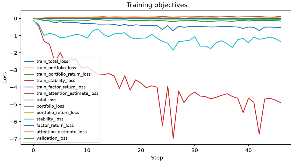
图 1 本次 CSI500 Fold 0 训练目标与验证损失曲线
