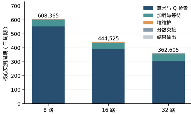
图 5: 同一预训练权重派生 H32/N640/K512 输入下, 运算通道数对核心周期数的影响。全部得分和选择结果一致。该核心独立测试不包含封装层的位置排序及原生 DMA / 存储等待; 结果输出周期取决于测试平台的 ready 序列。不同实现之间不预设时钟频率或 PPA 等价。
